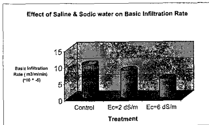
شکل ۲- تغییرات نفوذپذیری نهایی خاک تحت تأثیر کیفیت‌های مختلف آب آبیاری در آخر دوره
